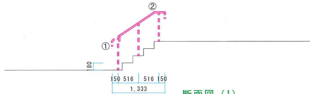
断面図 (1)
