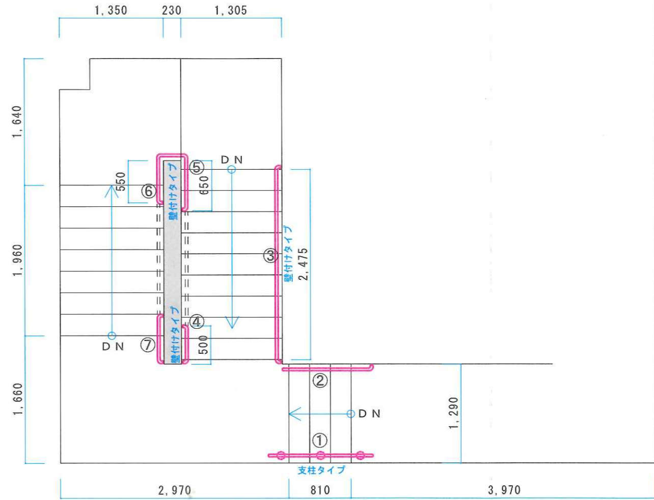
平面図 S = 1/50
