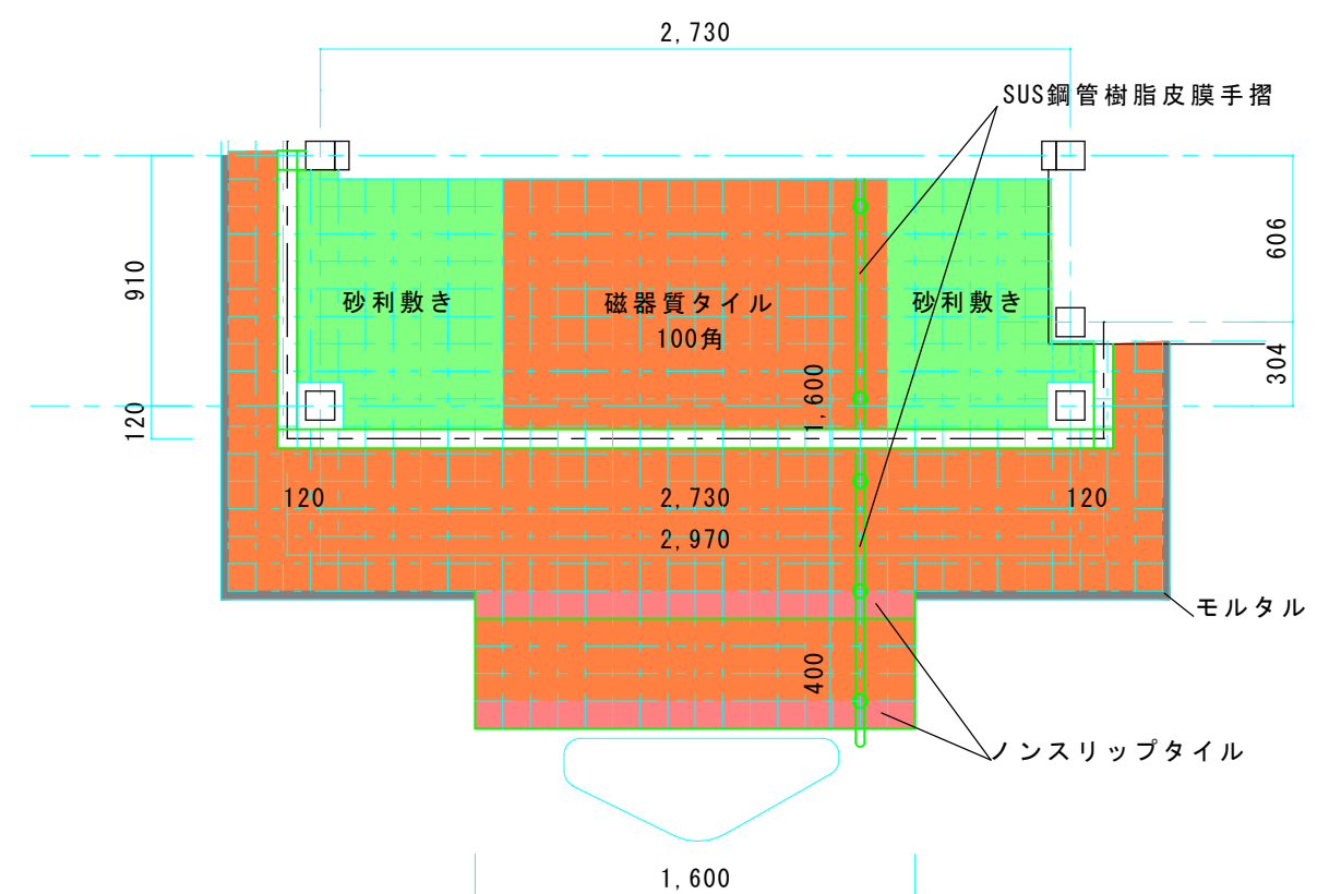
改修平面図 S = 1/30
