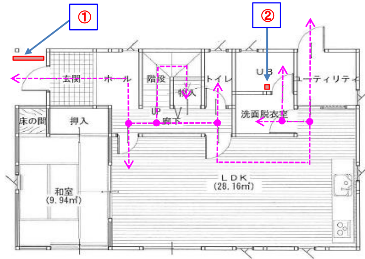
1階 平面図 S:1/100
