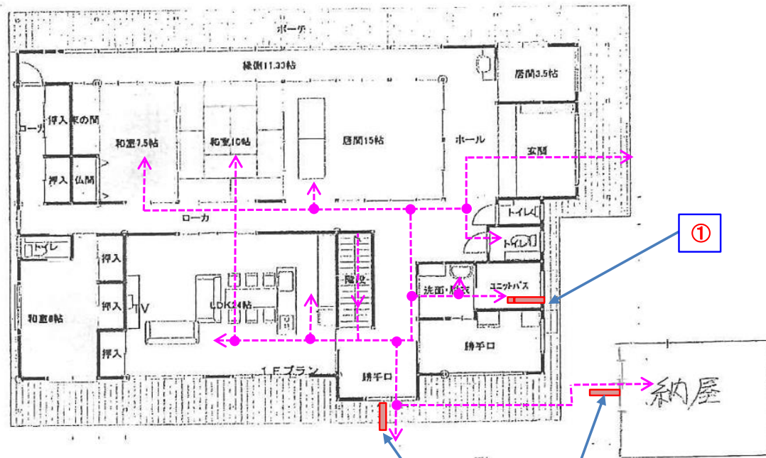
1階平面図 S:1/150
